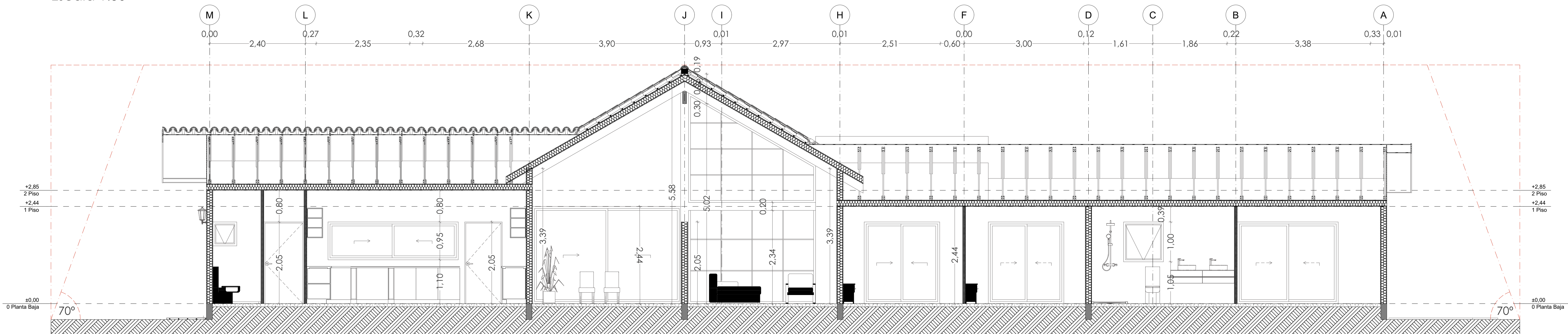
CORTE D-D Escala 1:50
