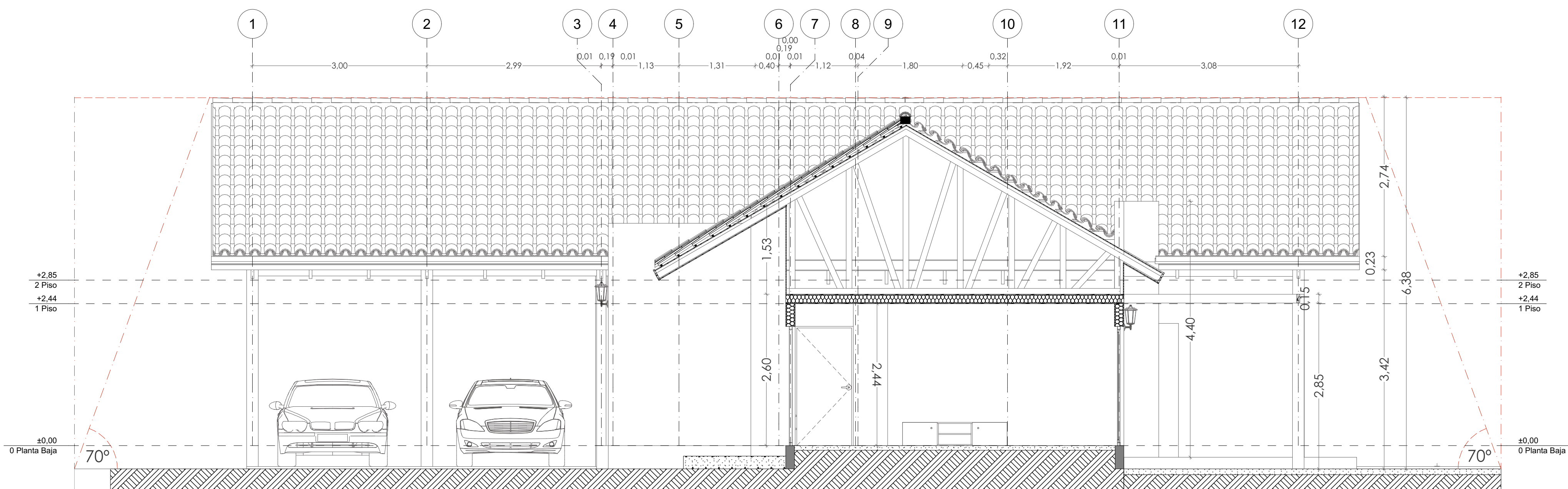
CORTE E-E Escala 1:50
